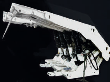
GIÀN CHỐNG CƠ KHÍ HÓA
